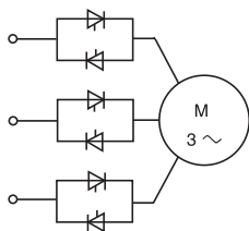
Принципиальная схема
