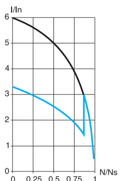
Пусковой ток
