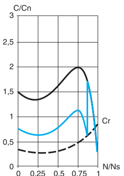
Пусковой момент
